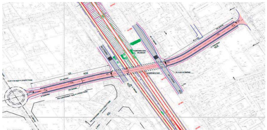
Projekt tunelu drogowego w Falenicy. Źródło: prezentacja PKP PLK S.A.
