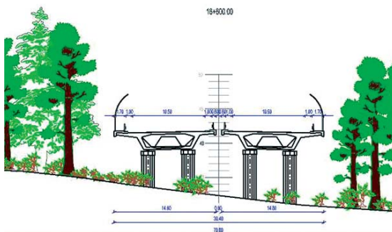
Filary estakady w Mazowieckim Parku Krajobrazowym
