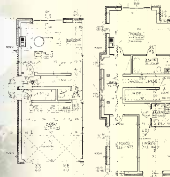
Rzut parteru
