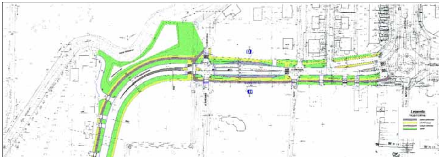
Projektowane rozwiązania komunikacyjne ulicy Nowoborkowskiej, od Ronda Graniczna do Cyraneczki (KomProjekt s.c.)
