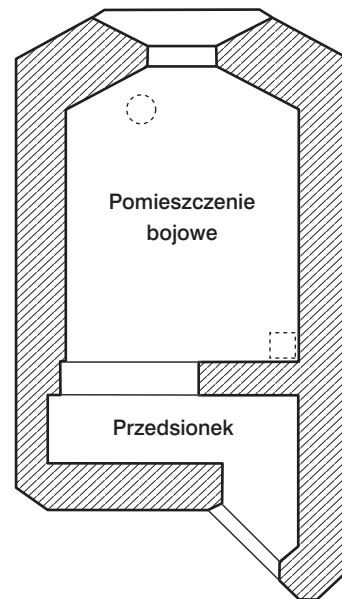
Rzut poziomy schronu spod Zagórze
