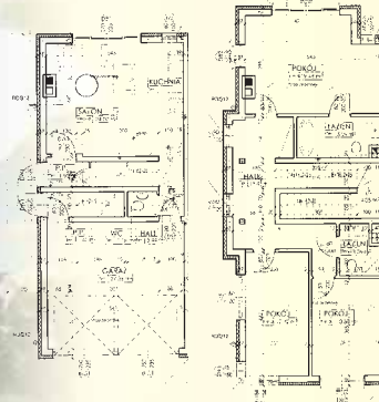
Rzut parteru
